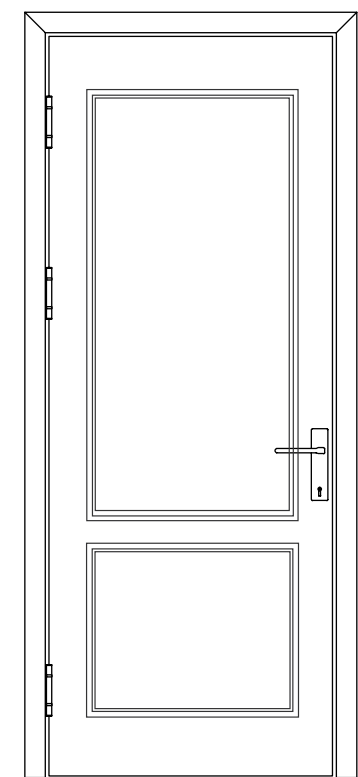
Bản vẽ bộ cửa điển hình
